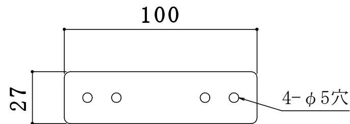
※HTL矢視図
